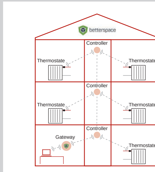
86 Funktionsprinzip iQ Roomcontrol von Betterspace GmbH
