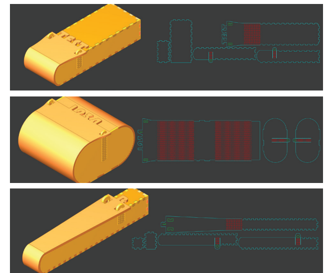
Mögliche Variationen der Schachtel inklusive 3D Visualisierung (links) und Schnittdatei für Lasercutter (rechts)
