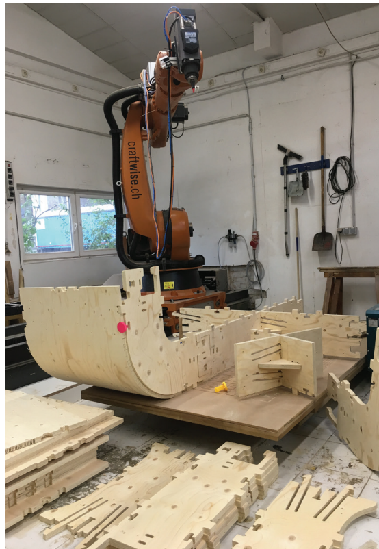
Digitale Fabrikation mit Hilfe eines 7-achsigen KUKA Industrieroboter
